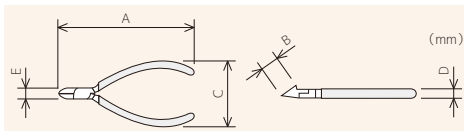
刃断面
