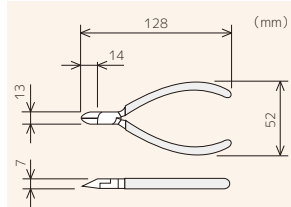
刃断面
